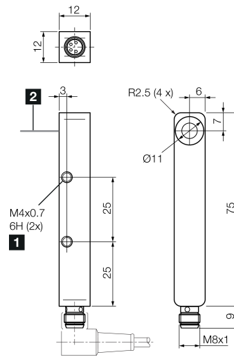
1) Bohrung / Gewinde (durchgehend) / Boring / thread (continuous) / Alésage / Filetage (traversant) 2) Schallaustritt Ultraschallwandler / Sound outlet ultrasonic transducer / Sortie sonore transducteur à ultrasons mm
