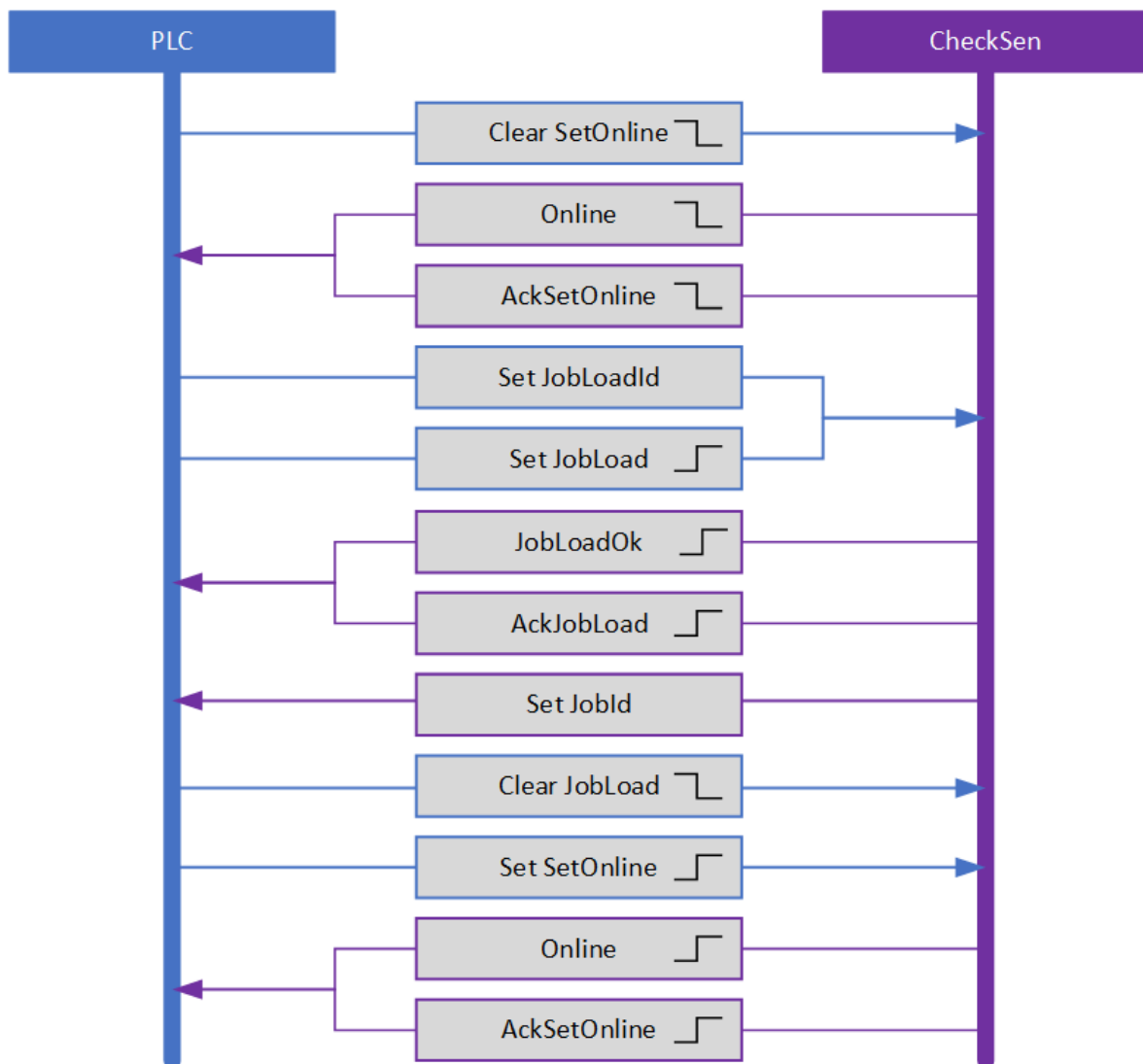
Abb. 162: Die JobLoad Sequenz
