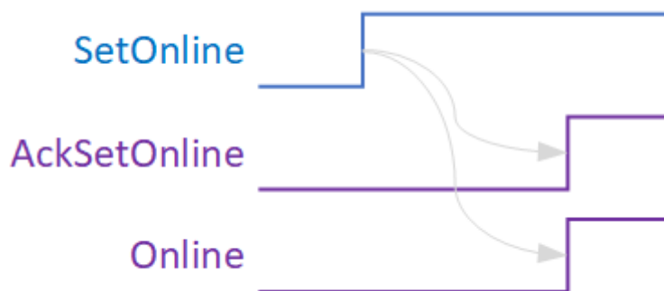
Abb. 160: Das SetOnline Zeitverhalten.
