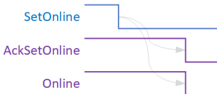
Abb. 161: Das SetOffline Zeitverhalten.
