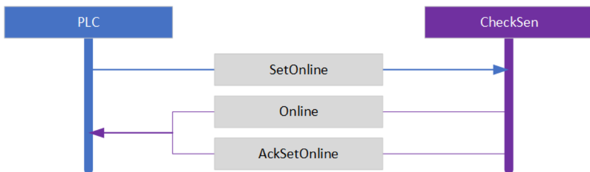
Abb. 159: Die SetOnline Sequenz
