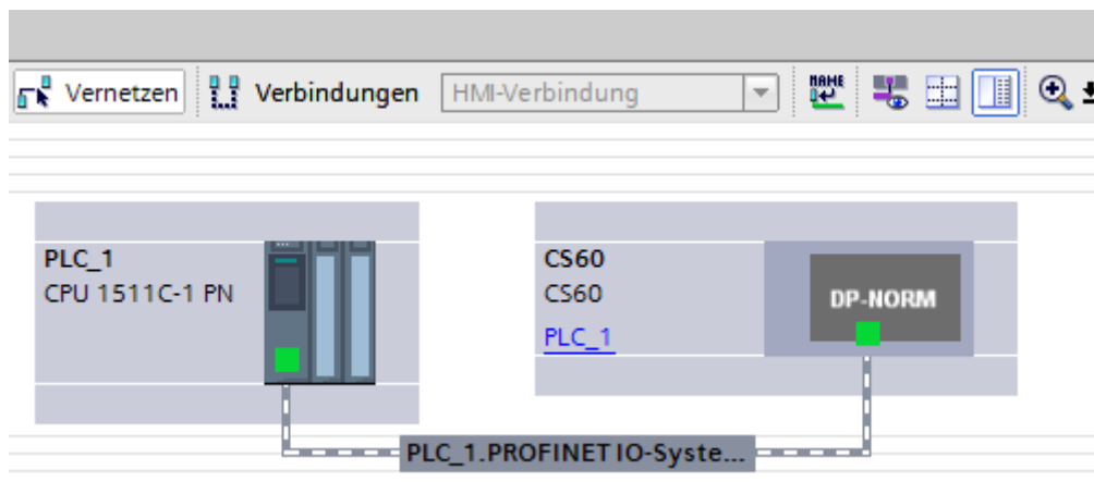
Abb. 151: Verbindung der SPS mit dem CS-60/ID-600
