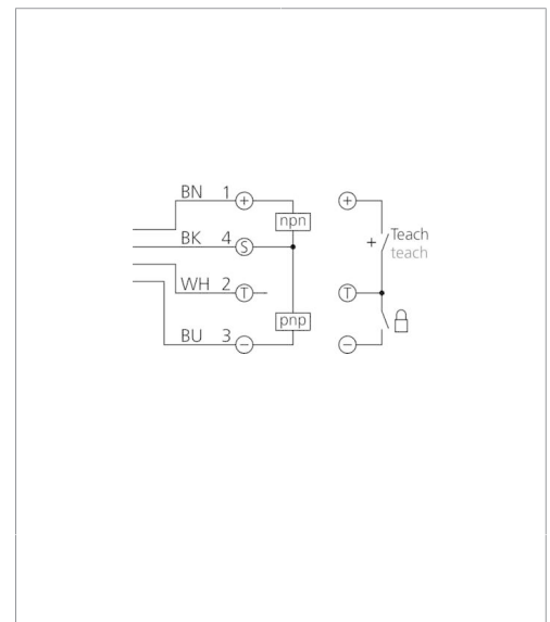
BK : schwarz / black / noir BU : blau / blue / bleu BN : braun / brown / marron WH : weiß / white / blanc
