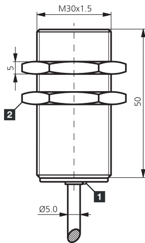
1) LED 2) Schlüsselweite 36 mm BK: schwarz BN: braun BU: blau
