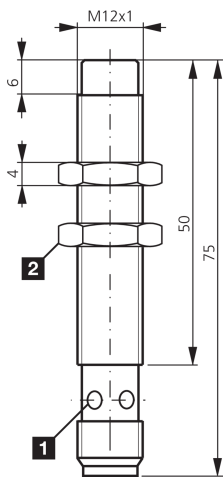
1) LED 4 x 90° (gelb) 2) Schlüsselweite 17 mm
