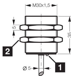
1) LED 2) Schlüsselweite 36 mm BK: schwarz BN: braun BU: blau
