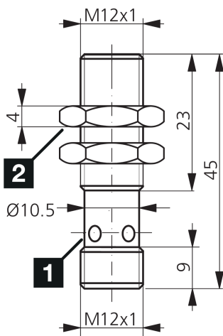
1) LED 4 x 90° (gelb) 2) Schlüsselweite 17 mm BK: schwarz BN: braun BU: blau
