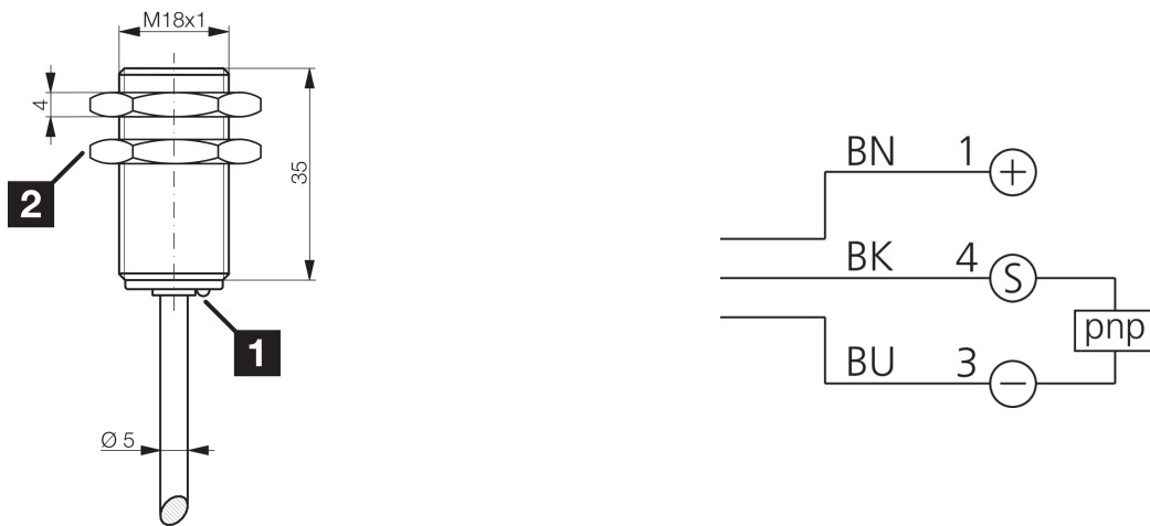
1) LED 2) Schlüsselweite 24 mm BK: schwarz BN: braun BU: blau
