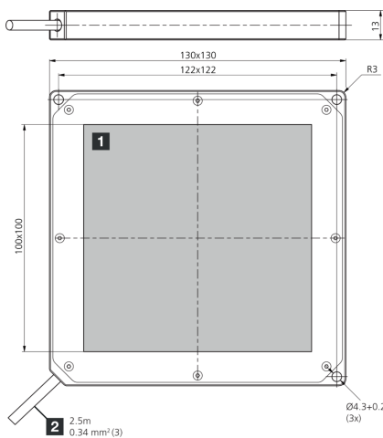
2) Anschlusskabel
