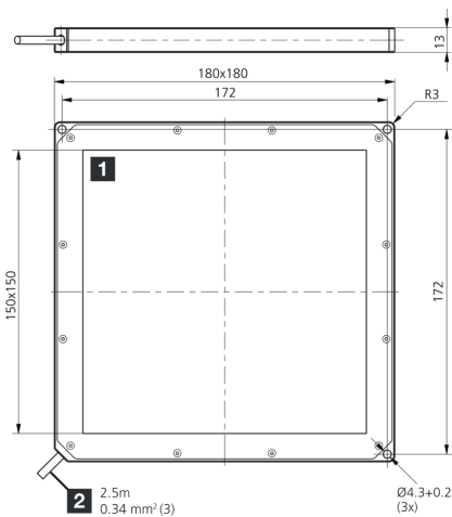
2) Anschlusskabel
