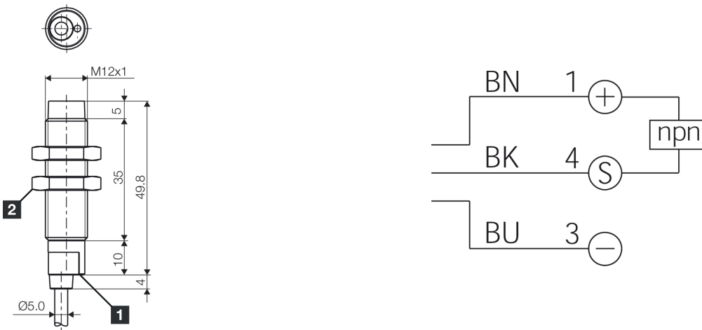
1) LED 2) Schlüsselweite 17 mm BK: schwarz BN: braun BU: blau
