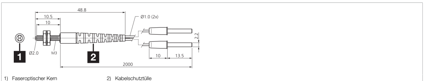
1) Faseroptischer Kern
