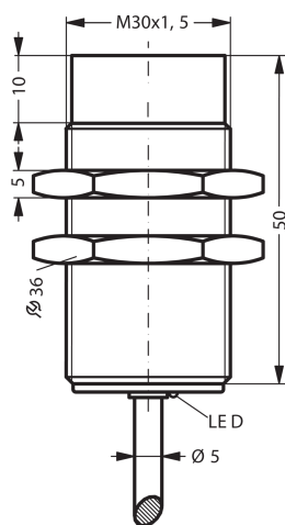
2) Width over flats 36 mm
