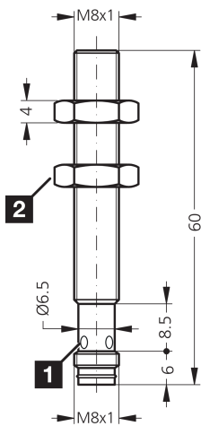
1) LED 4 x 90° (jaune) 2) Ouverture de clé 13 mm BK: noir BN: marron BU: bleu
