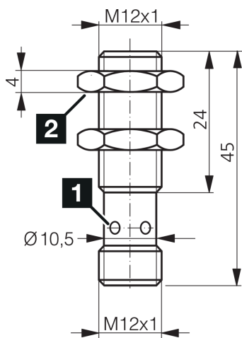
1) LED 4 x 90° (jaune) 2) Ouverture de clé 17 mm BK: noir BN: marron BU: bleu
