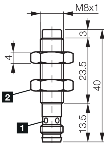
1) LED 4 x 90° (jaune) 2) Ouverture de clé 13 mm BK: noir BN: marron BU: bleu
