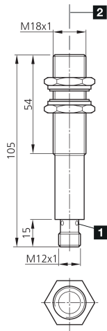
1) LED 4 x 90° (jaune) 2) Sortie sonore transducteur à ultrasons BK: noir BN: marron BU: bleu WH: blanc
