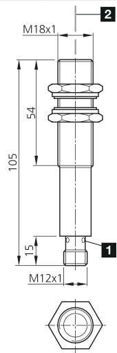
1) LED 4 x 90° (gelb) / LED 4 x 90° (yellow) / LED 4 x 90° (jaune) 2) Schallaustritt Ultraschallwandler / Sound outlet ultrasonic transducer / Sortie sonore transducteur à ultrasons mm
