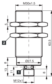
1) LED 4 x 90° (黄色) 2) 开口度 36 mm BK: 黑色 BN: 棕色 BU: 蓝色
