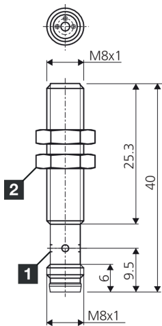
1) LED 2) 开口度 13 mm BK: 黑色 BN: 棕色 BU: 蓝色
