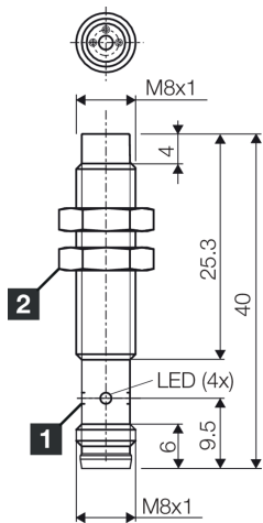
1) LED 4 x 90° (黄色) 2) 开口度 13 mm BK: 黑色 BN: 棕色 BU: 蓝色
