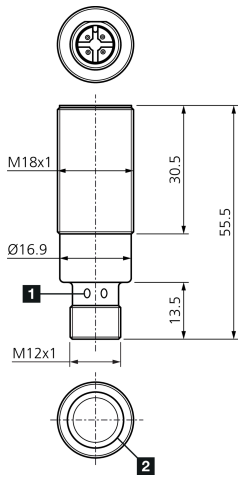
1) LED 2 x 2 2) 超声波换能器声出口 BK: 黑色 BN: 棕色 BU: 蓝色 WH: 白色
