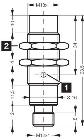
1) LED 2) Schlüsselweite 24 mm BK: schwarz BN: braun BU: blau
