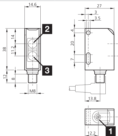
1) Potentiometer / Potentiometer / Potentiomètre 2) Optische Achse (E) / Optical axis (R) / Axe optique (R) 3) Optische Achse (S) / Optical axis (T) / Axe optique (È) mm
