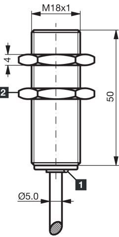
1) LED 2) 开口度 24 mm BK: 黑色 BN: 棕色 BU: 蓝色
