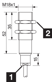
1) LED 2) 开口度 24 mm BK: 黑色 BN: 棕色 BU: 蓝色
